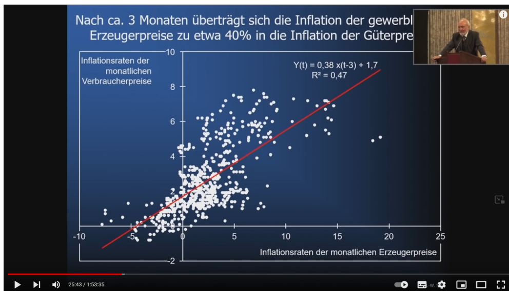
Abbildung 9.3: Problematische Anwendung der Regression und des Bestimmtheitsmaß [3]
