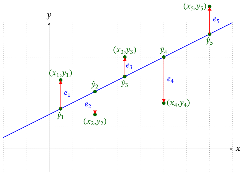
Abbildung 9.1: Einzelfehler bei Anpassung einer Gerade
