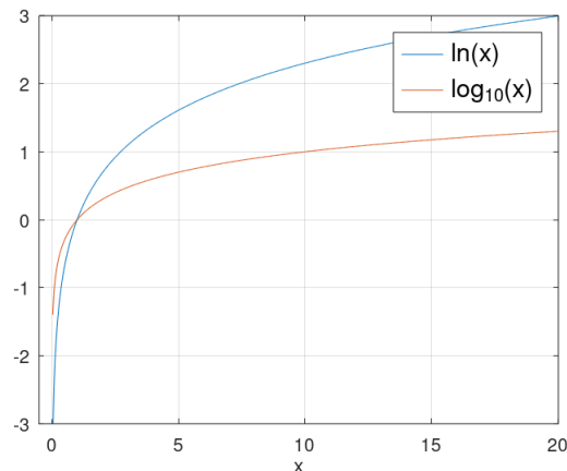
Dekadischer \log_{10}(x) und natürlicher \ln(x) Logarithmus
