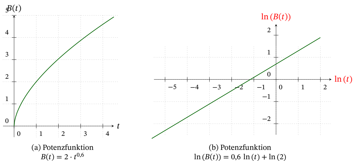
Abbildung 9.5: Darstellung Potenzfunktion normal und doppellogarithmisch
