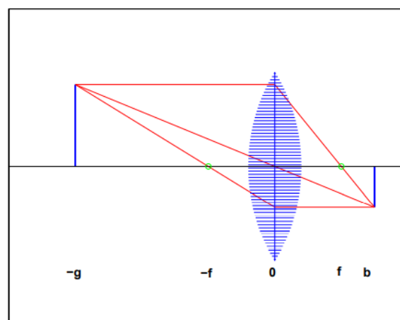
Abbildung 6.3: Sammellinse
