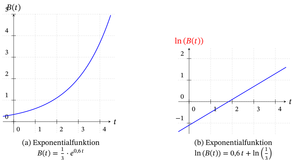
Abbildung 9.4: Darstellung Exponentialfunktion normal und semilogarithmisch
