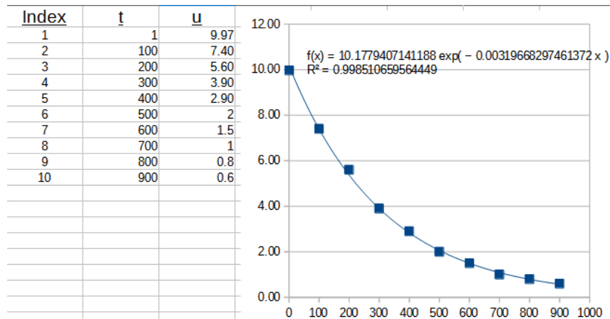
Abbildung 15.1: Lösung Exponentialfunktion
