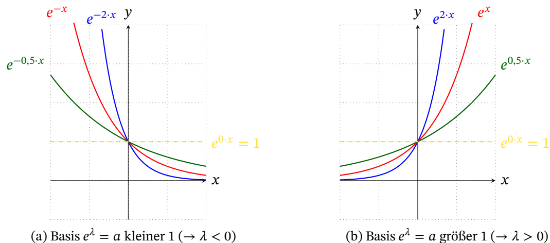
Abbildung 7.2: Exponentialfunktion e^{\lambda x}
