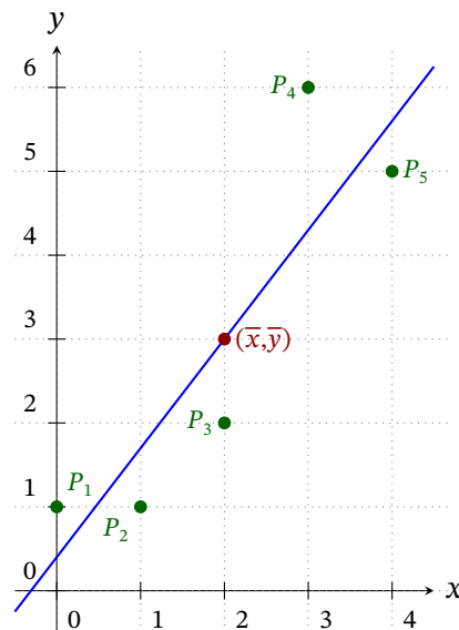
Abbildung 9.2: Einzelfehler bei Anpassung einer Gerade
