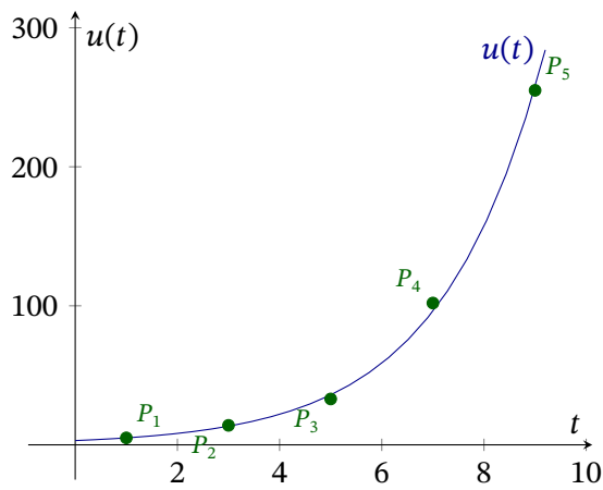
(a) Exponentialgesetz u(t) = 3,06 \cdot e^{0,4925 \cdot t}
