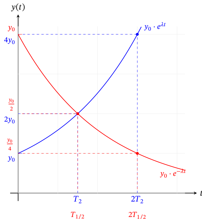
Abbildung 8.2: Vergleich von Wachstum und Zerfall: Nach jeweils einem weiteren Intervall T_2 bzw. T_{1/2} hat sich der Wert erneut verdoppelt bzw. halbiert.
