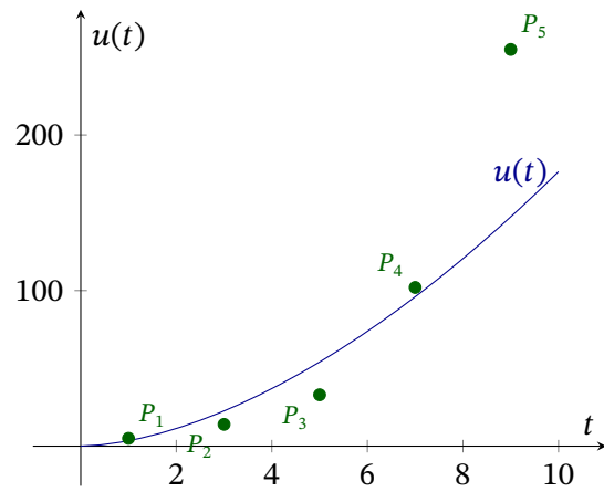
(b) Potenzgesetz u(t) = 3,47 \cdot t^{1,7062}
