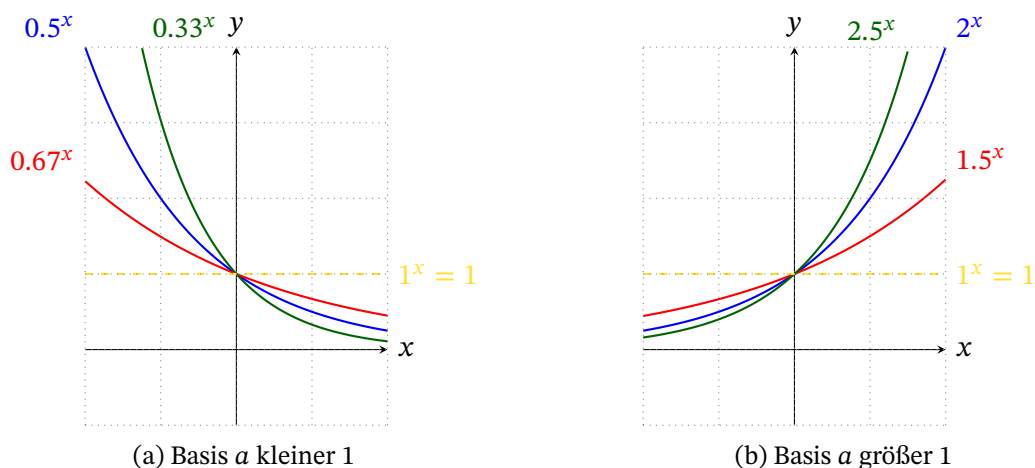
Abbildung 7.1: Exponentialfunktion a^x
