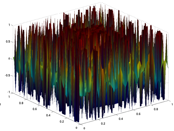
(d) dual solution p
